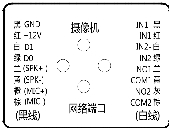
指纹仪背面接线端口图
